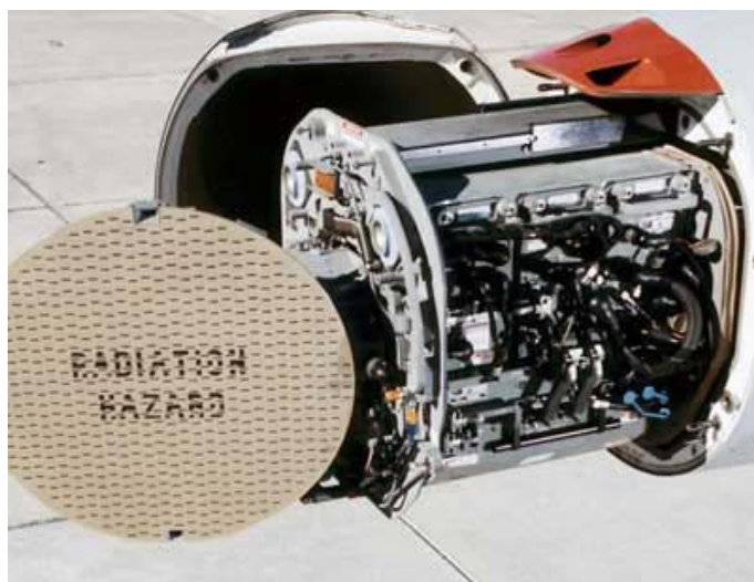
AN/APG-73 F/A-18C/D/E/F
